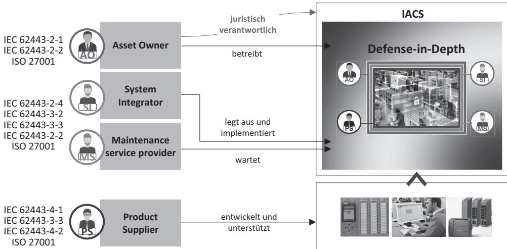
Bild 5.1 Tiefgestaffelte Verteidigung (Defense-in-Depth)
